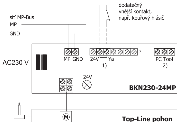
Obr. 23 Komunikační a napájecí zařízení BKN 230-24MP
