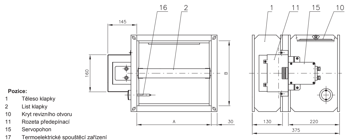
Obr. 29 PKTM 90 - C - provedení se servopohonem do (ZÓNA 1,2)
