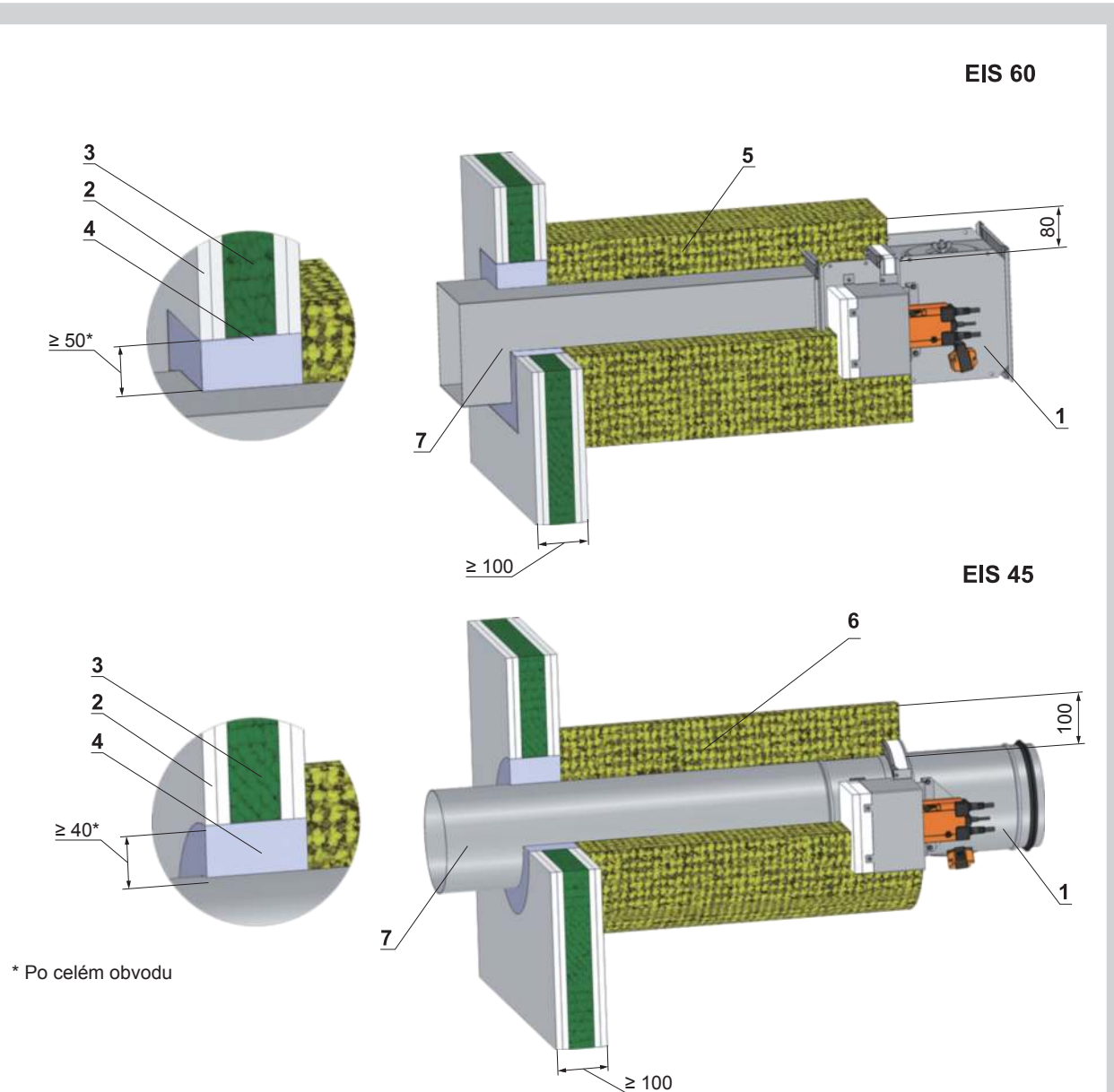
Obr. 59 Mimo tuhou stěnovou konstrukci - doizolace minerální vlnou
