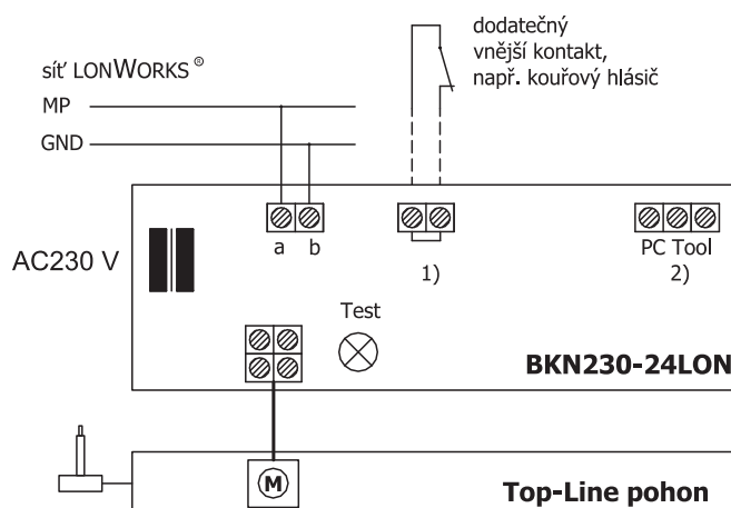
Obr. 24 Komunikační a napájecí zařízení BKN 230-24LON
