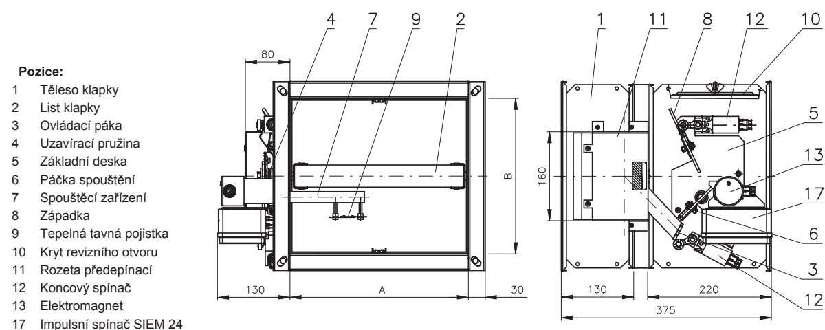
Obr. 28 PKTM 90 - C - provedení se servopohonem
