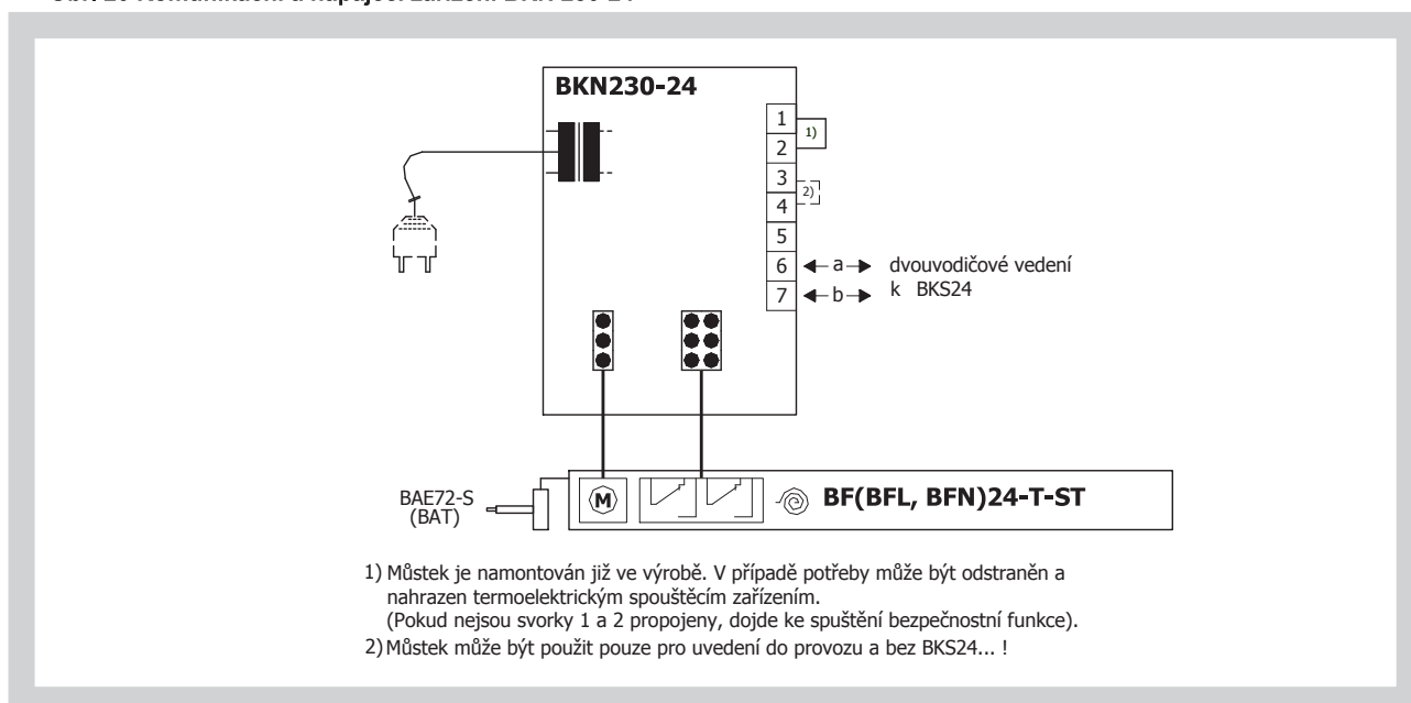
Obr. 20 Komunikační a napájecí zařízení BKN 230-24
