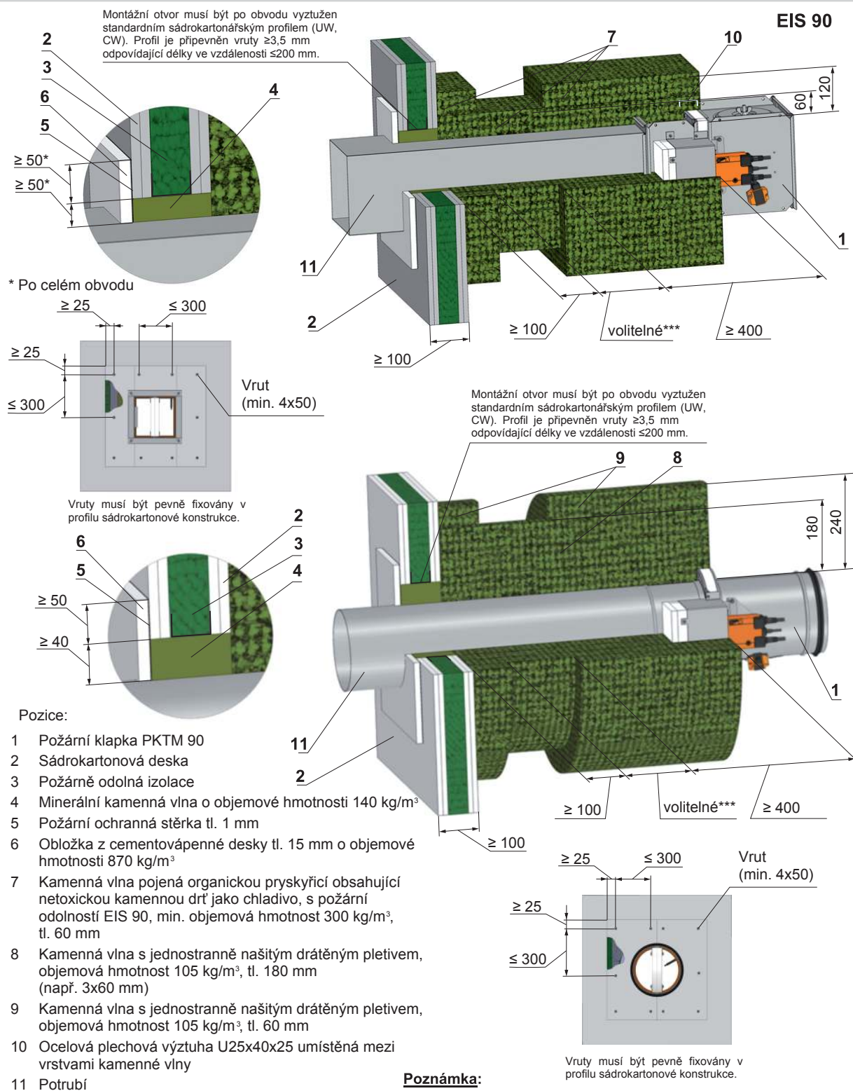
Obr. 52 Mimo sádrokartonovou konstrukci - doizolace minerální vlnou
