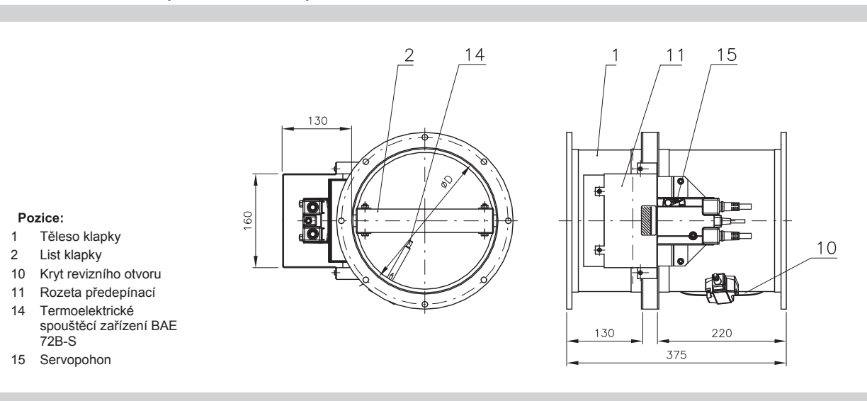
Obr. 31 PKTM 90 - K - provedení se servopohonem
