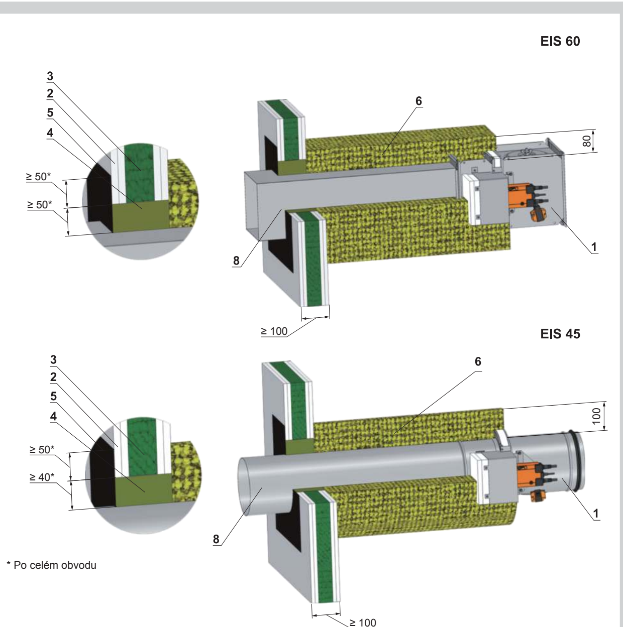
Obr. 60 Mimo tuhou stěnovou konstrukci - doizolace minerální vlnou
