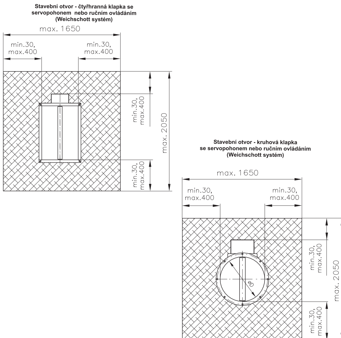
Obr. 39 Doporučené stavební otvory - Weichschott system
