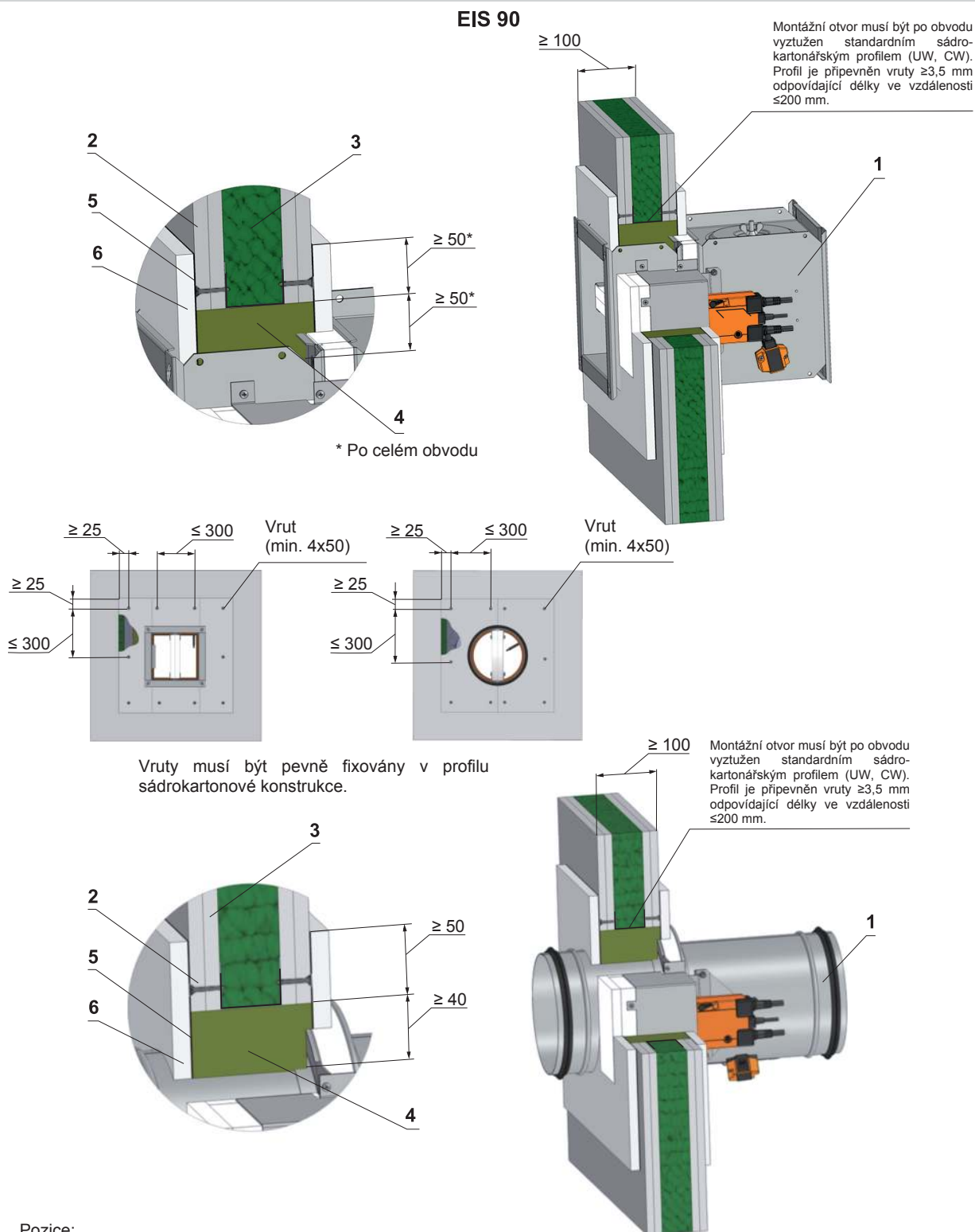
Obr. 50 Sádkartonová konstrukce - požární ucpávka se stěrkou a cementovápennými obložkami
