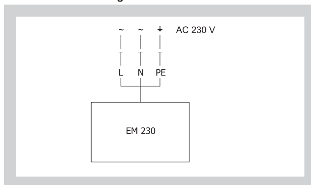
Obr. 7 Elektromagnet EM230
