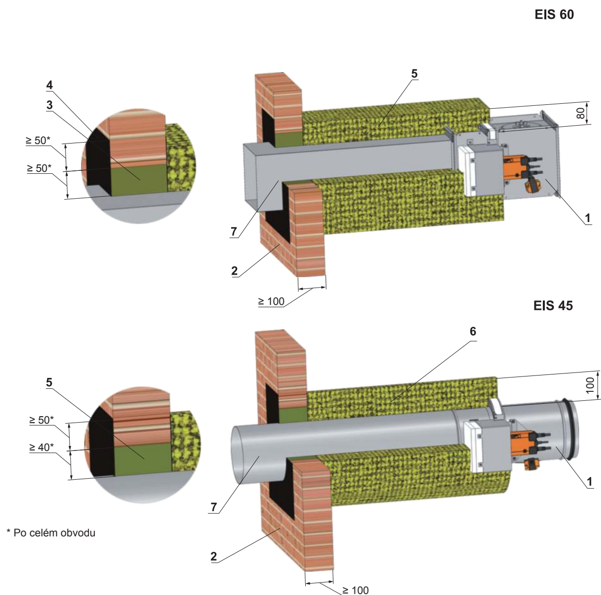
Obr. 58 Mimo tuhou stěnovou konstrukci - doizolace minerální vlnou
