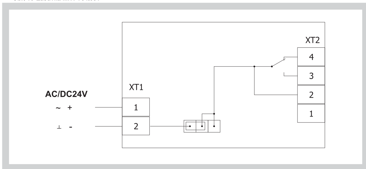
Obr. 16 Zásuvka MHY 734.031
