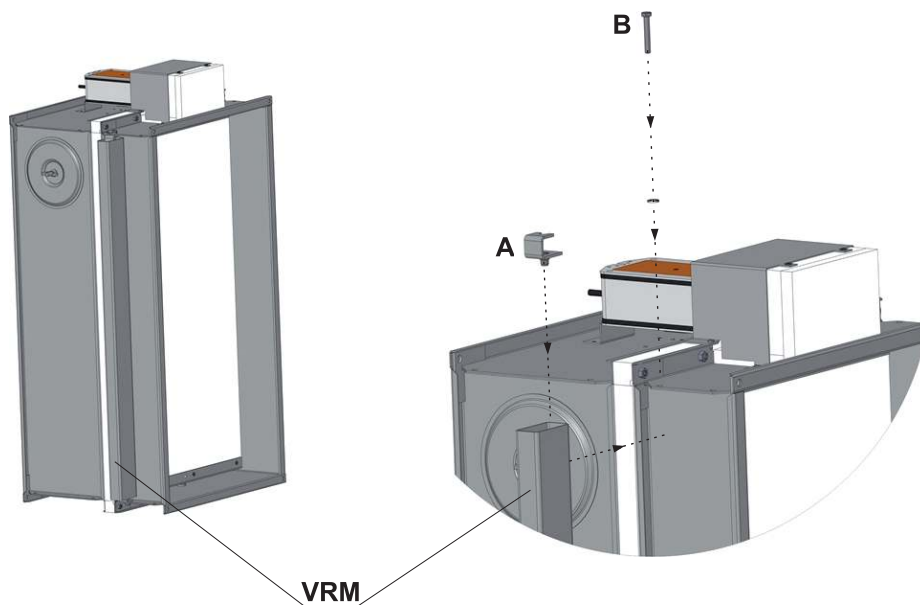
Obr. 53 Upevnění vyztužovacího rámu na čtvercovou klapku v případě umístění mimo stěnovou nebo stropní konstrukci
