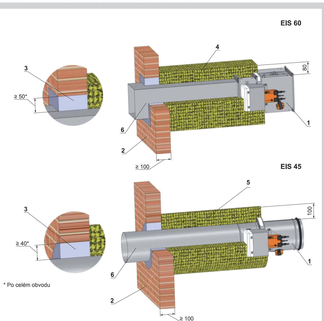
Obr. 57 Mimo tuhou stěnovou konstrukci - doizolace minerální vlnou
