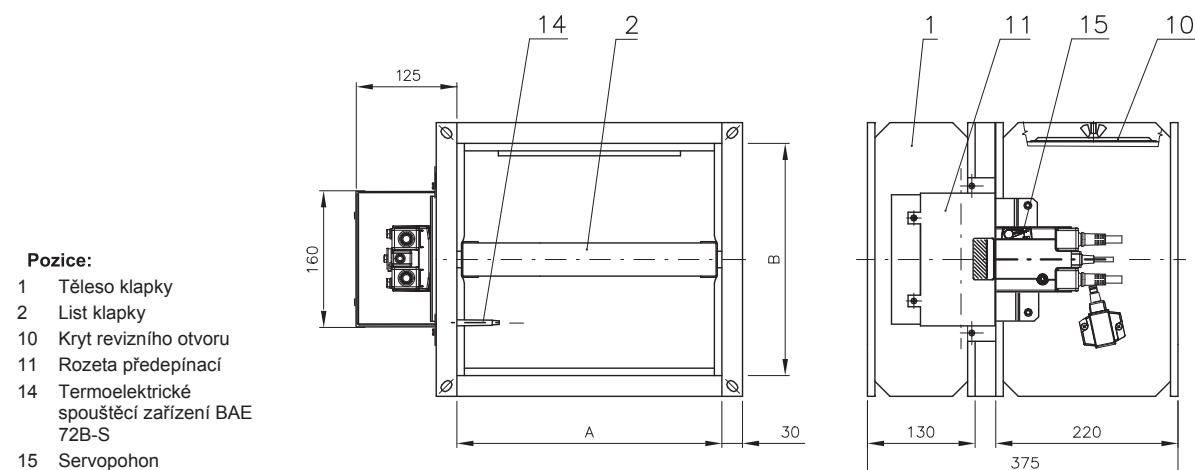
Obr. 29 PKTM 90 - C - provedení se servopohonem do (ZÓNA 1,2)
