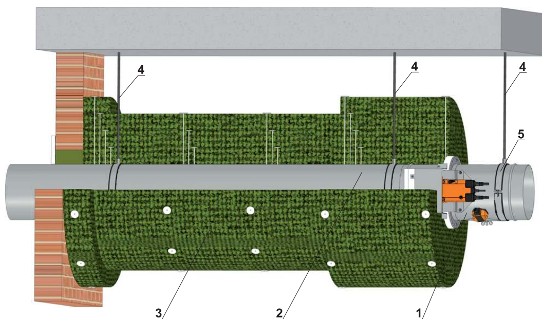
Obr. 67 Příklady zavěšení kruhových klapek na stěnu - vodorovná instalace
