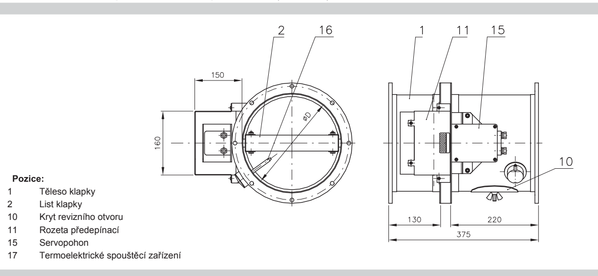
Obr. 32 PKTM 90 - K - provedení se servopohonem do (ZÓNA 1,2)
